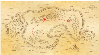
Geländesuchspiel
